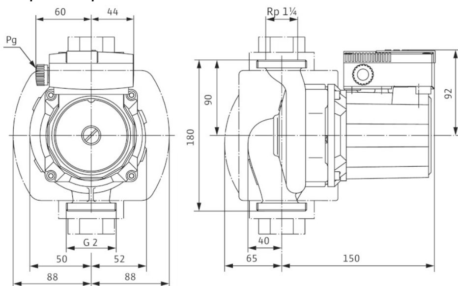
Габаритный чертеж
