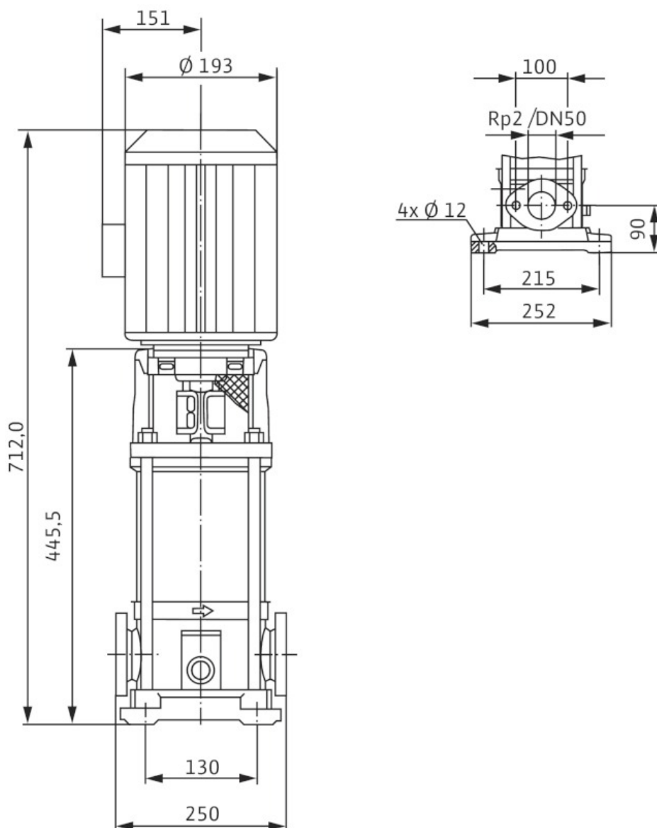
Габаритный чертеж
