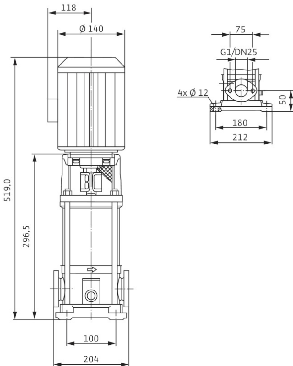
Габаритный чертеж
