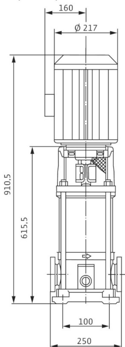
Габаритный чертеж
