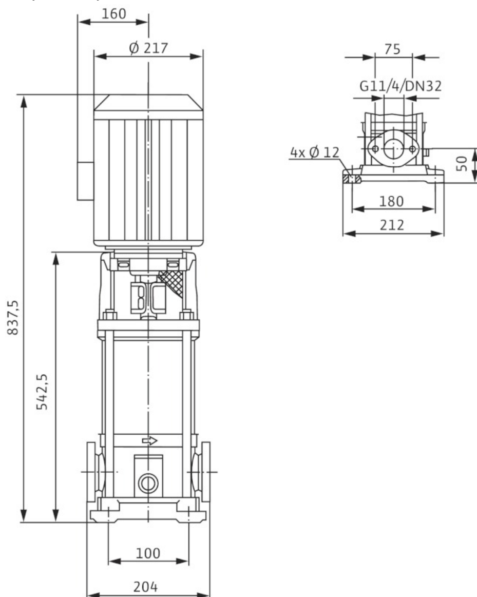
Габаритный чертеж
