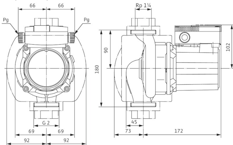
Габаритный чертеж
