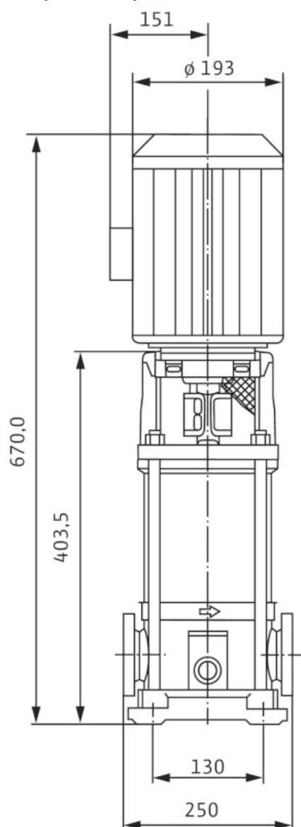
Габаритный чертеж
