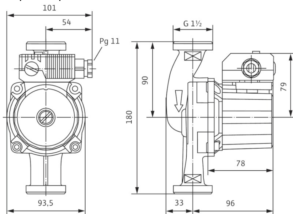
Габаритный чертеж
