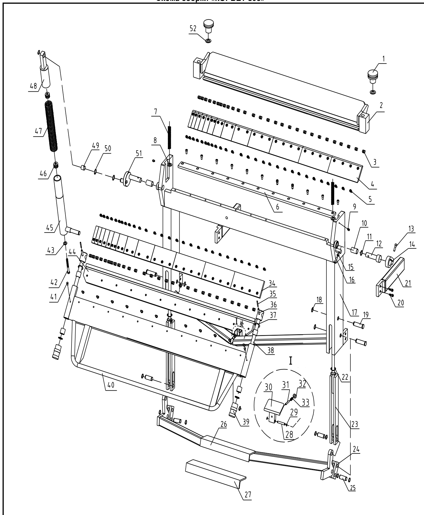
Схема сборки «КОРВЕТ 506»
