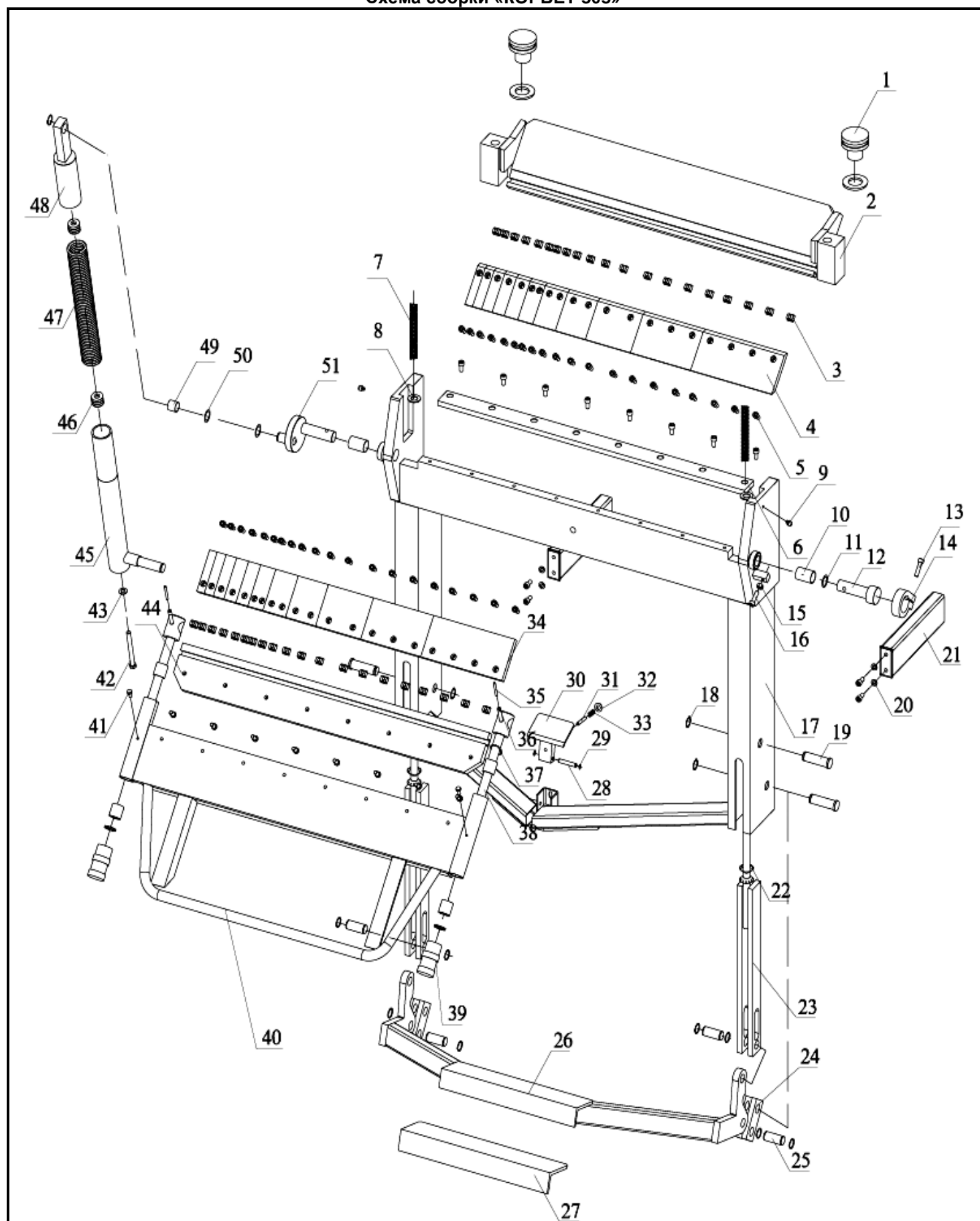
Схема сборки «КОРБЕТ 505»
