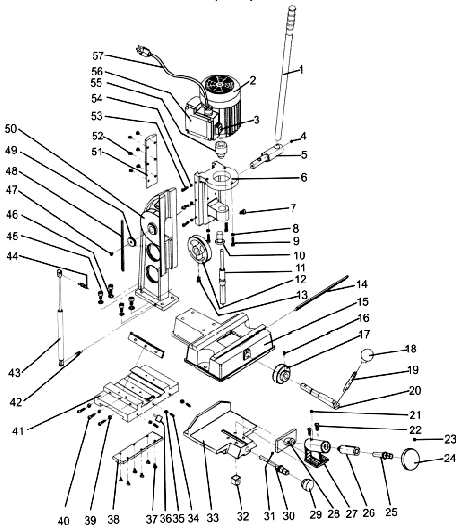
Схема сборки «Корвет 91»
