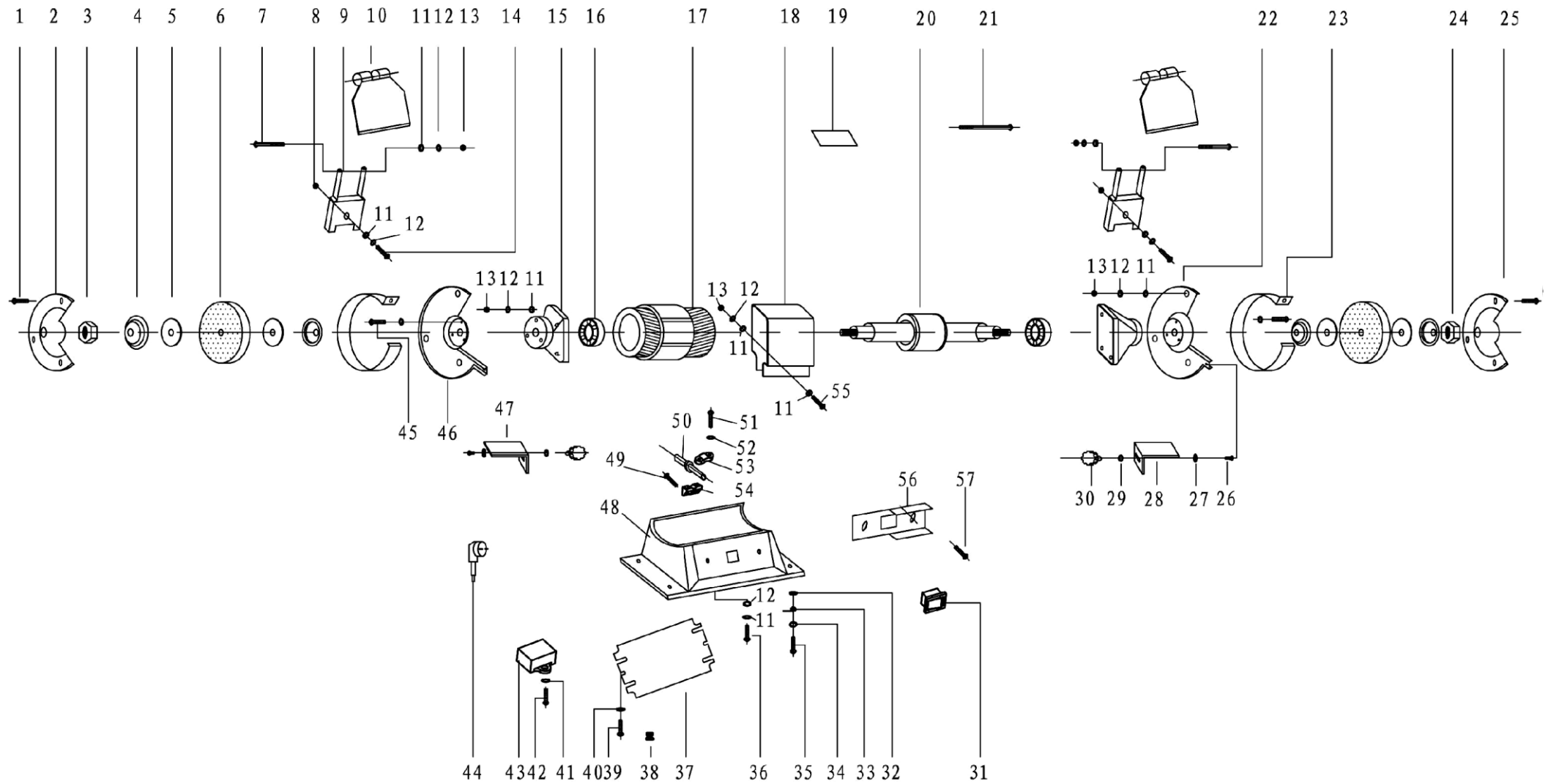
Схема сборки «КОРВЕТ 486»
