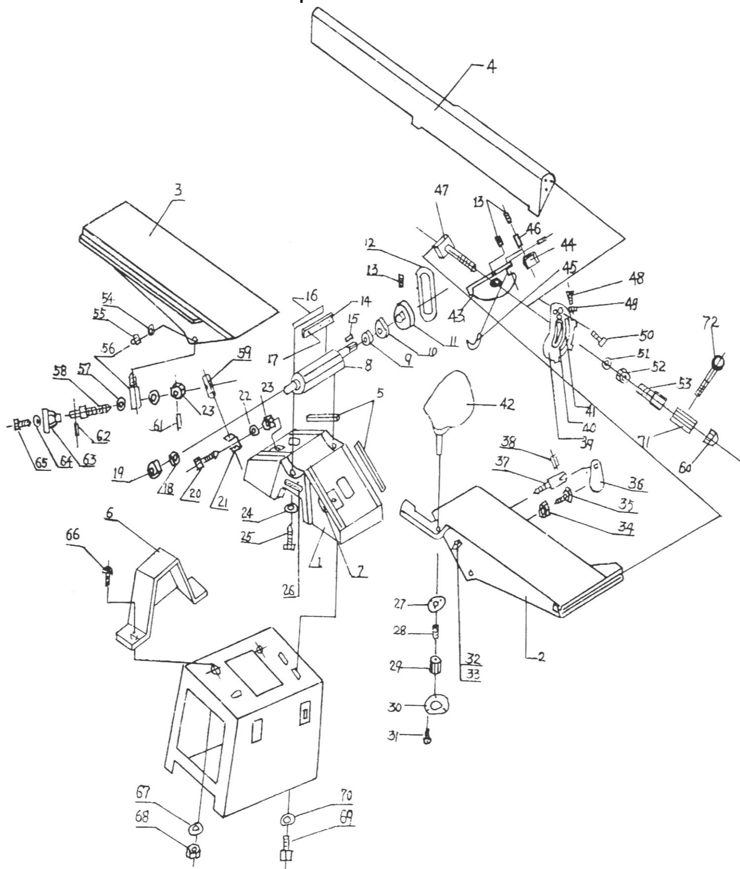
Схема сборки машины «КОРВЕТ 106»
