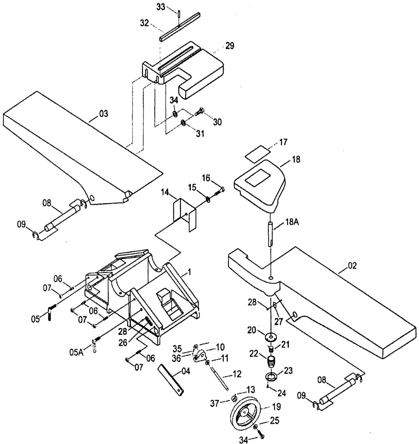
Схема сборки машины «КОРВЕТ 104»
