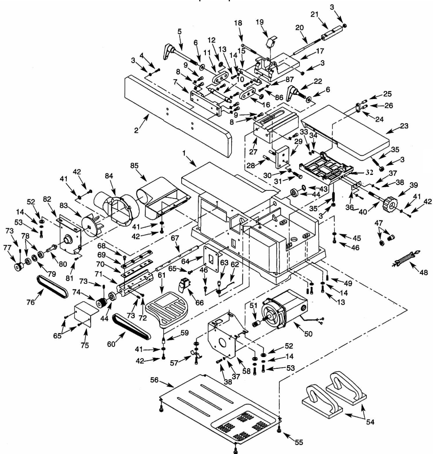
Схема сборки «Корвет 101»
