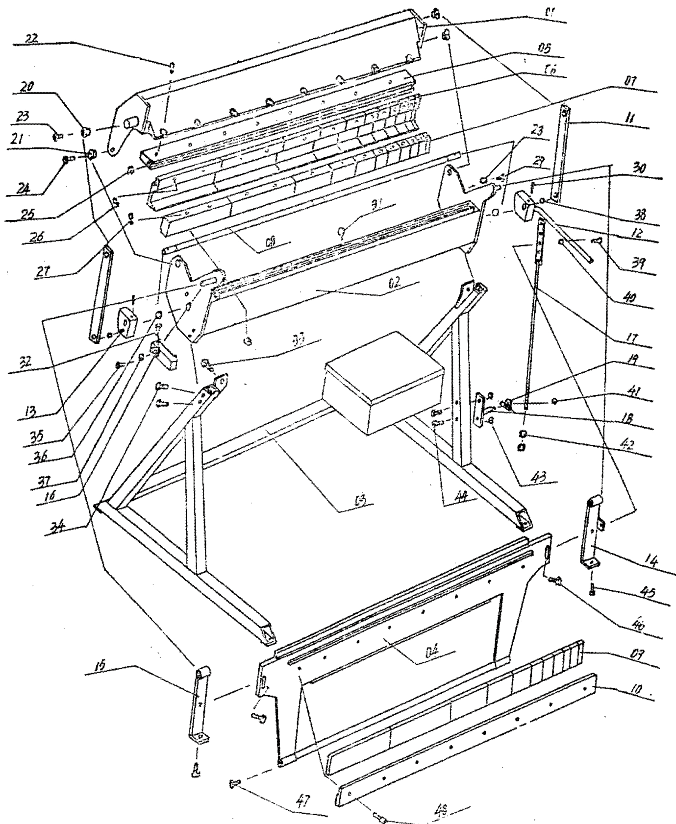
Схема сборки «КОРВЕТ 504»
