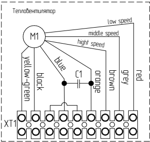
Внутреннее устройство клеммной коробки: XT1 – клеммная колодка; C1 – конденсатор; M1 – электродвигатель; Расцветка выводных проводов электродвигателя: Yellow-green (желто-зеленый) – провод заземления; Black, orange (черный, оранжевый) – провода нейтрал; Brown (коричневый) – провод максимальной скорости; Grey (серый) – провод средней скорости; Red (красный) – провод минимальной скорости.
