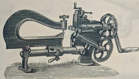
№ 2. Ножницы для вырѣзызанія кружковъ и полосъ
