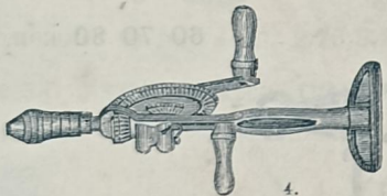
№ 4. Коловоротъ аме- риканскій большой для сверленія дерева и ме- талла.
