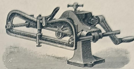
№ 1. Зикенъ машина
