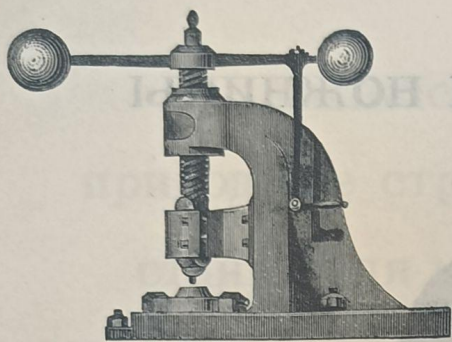
№ 1. Винтовые прессы боевые, чугунные, прочной конструкціи съ маховикомъ; по желанію можно имѣть ихъ съ балансомъ.
