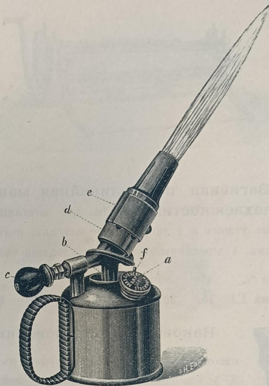
№ 35. Шведская бензиновая паяльная лампа
