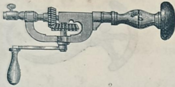
№ 2. Коловороты съ шестернями и боковой ручкой.
