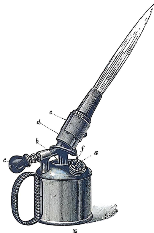
№ 35. Шведская бензиновая паяльная лампа
